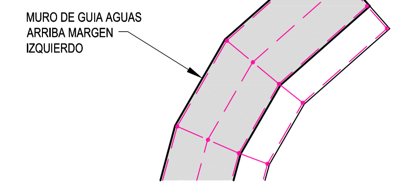
PAT MURO DE GUIA AGUAS ARRIBA DETALLE "A" ESC. 1:750
